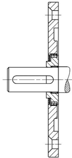
Motor B3/B5 und B3/B4
