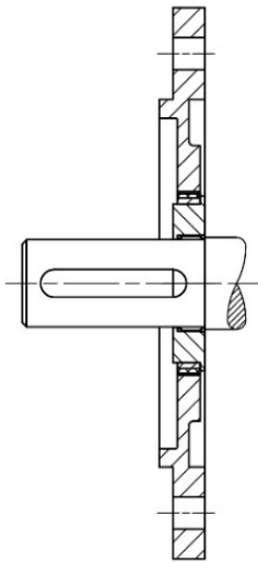
Motor B5 und B 14
