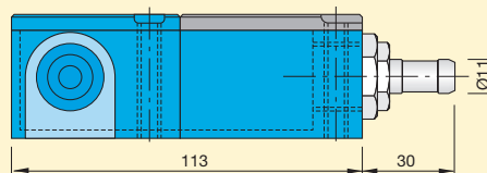
VERSIONE CON USCITA A CAVO VISTA LATERALE (IP67) VERSION WITH CABLE EXIT - SIDE VIEW
