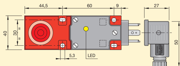
VERSIONE CON USCITA A CONNETTORE - VISTA SUPERIORE VERSION WITH CONNECTOR K - TOP VIEW
