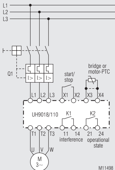
Softstart- and softstop function at UH 9018/110
