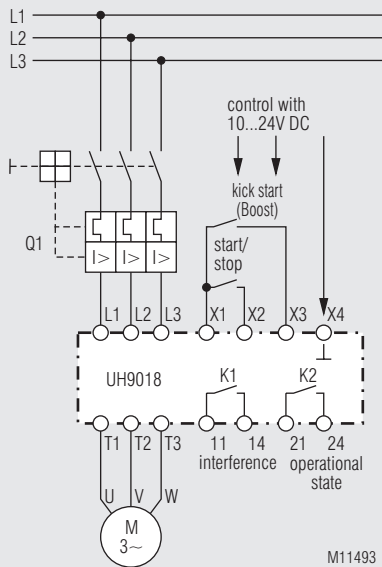
Softstart- and softstop function
