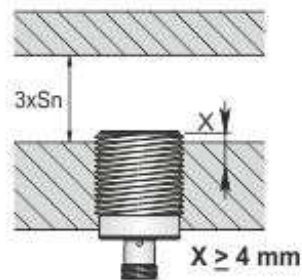
Montaggio a filo
