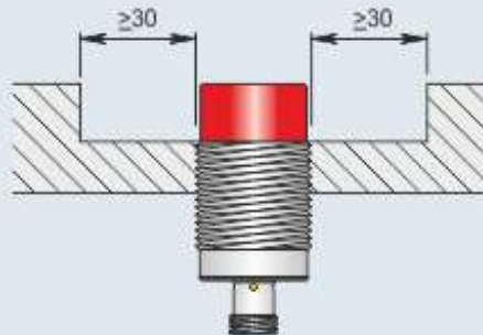
Montaggio sporgente
