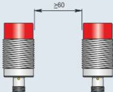
Montaggio affiancato
