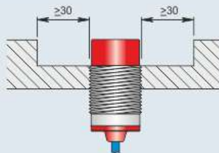
Montaggio sporgente
