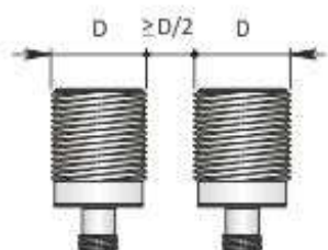
Montaggio affiancato
