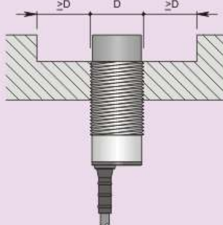
Montaggio sporgente
